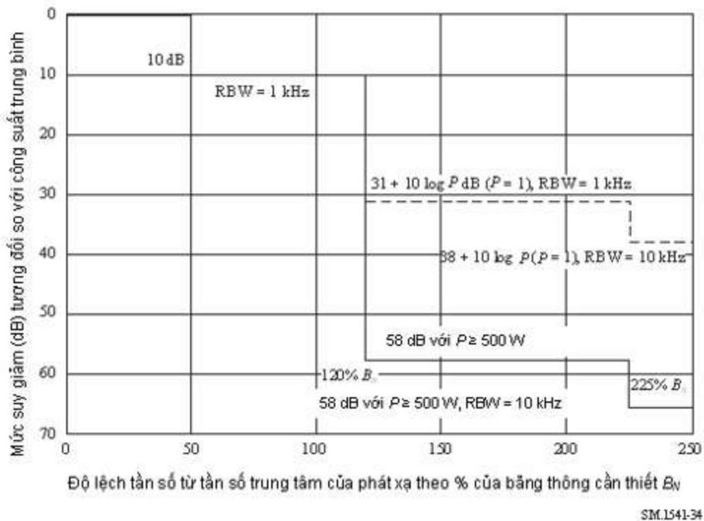
Hình D.10 - Các dải hoạt động trong dải tần trên 30 MHz trong trường hợp băng tiêu chuẩn hoặc băng hẹp của khuyến nghị ITU-R SM.1539
