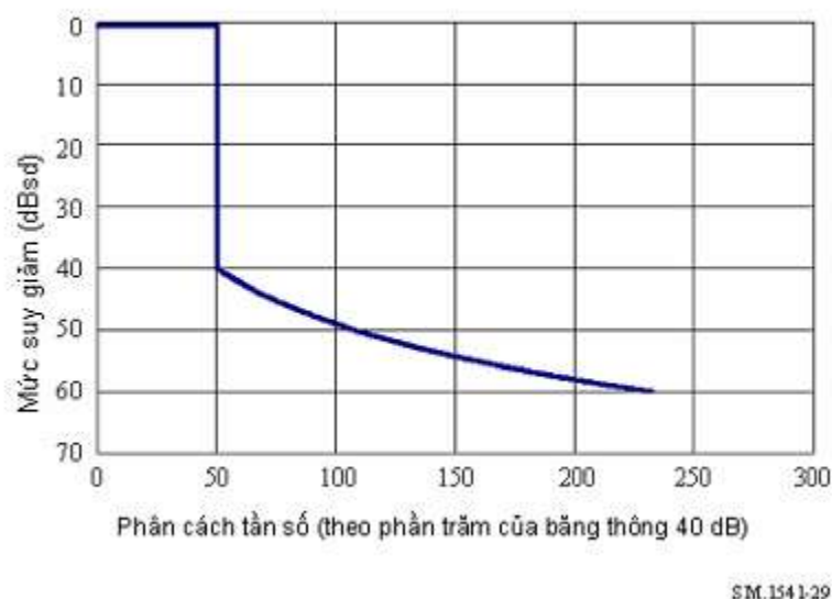
Hình D.6 - Mặt nạ phổ phát xạ ngoài băng đối với tất cả các dạng sóng ra-đa thuộc mục D.3.3 (không bao gồm các dạng sóng bị loại trừ ở mục D.3.4.2)
