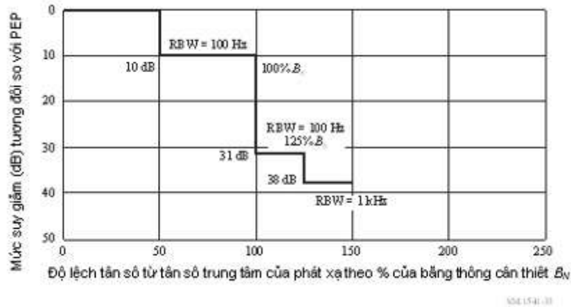
Hình D.9 - Các dải hoạt động trong dải tần dưới 30 MHz trong trường hợp băng rộng của khuyến nghị ITU-R SM.1539
