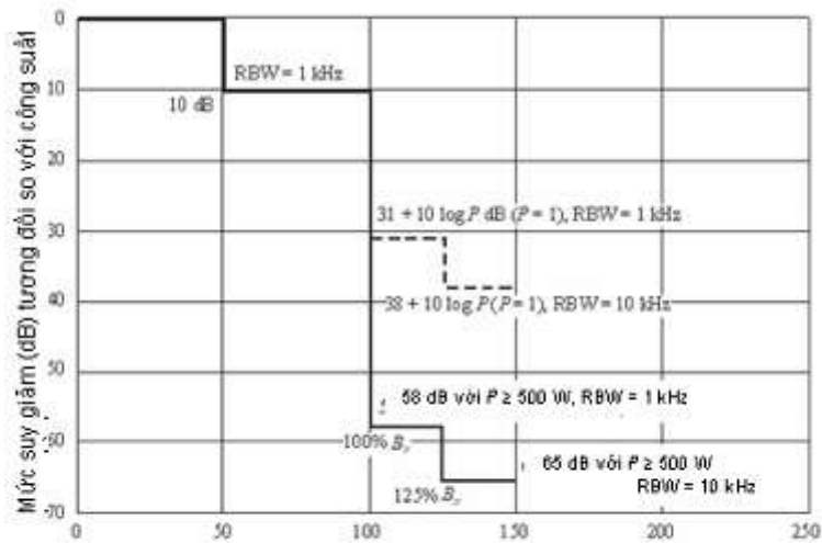
Độ lệch tần số từ tần số trung tâm của phát xạ theo % của băng thông cần thiết B_W
