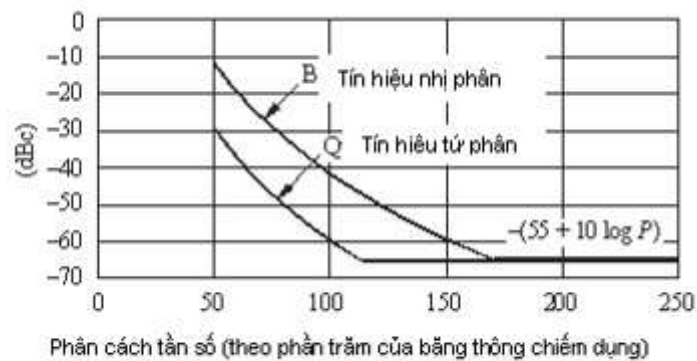
Hình D.15 - Ví dụ về mặt nạ phổ phát xạ ngoài băng cho đo đặc từ xa thuộc nghiệp vụ hàng không
