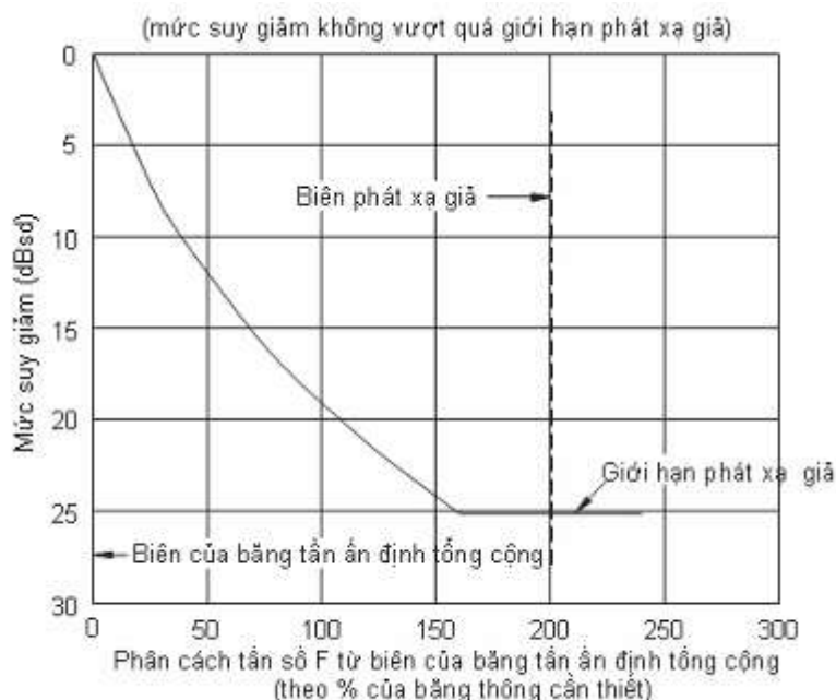
Hình D.2 - Ví dụ 1: Mật nạ phổ phát xạ ngoài băng với giả thiết giới hạn phát xạ giả tại điểm 25 dBsd
