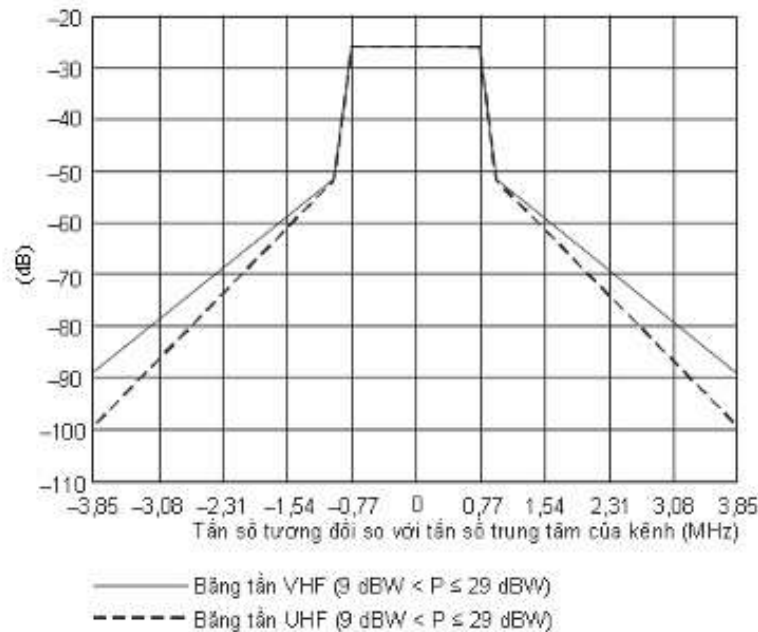
Hình D.5 - Mật nạ phổ phát xạ ngoài băng đối với hệ thống số loại A ( 9 \text{ dBW} < P \leq 29 \text{ dBW} )
