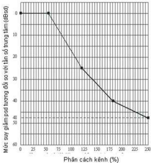
Hình D.18 - Mặt nạ phổ phát xạ ngoài băng cho nghiệp vụ cố định số hoạt động trong băng tần trên 30 MHz (xem Bảng D.8)
